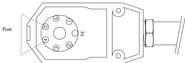
Fiche mâle EC
